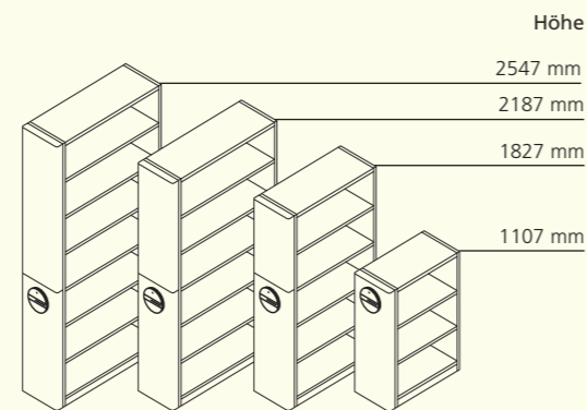
Erhältliche Regalbreiten 1200 mm, 1000 mm, 900 mm, 800 mm, 600 mm
