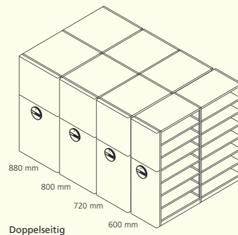
Erhältliche Regalbreiten 1200 mm, 1000 mm, 900 mm, 800 mm, 600 mm
